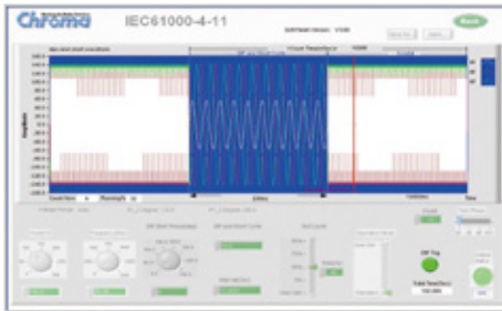
电压瞬断法规测试
