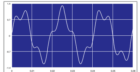
间谐波波形
